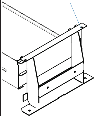
Fig 3 : Coloque el accesorio TROMEN® Lateral Pampeana sobre los agujeros de mensula lateral de su parrilla TROMEN®. Para un correcto ensamble
