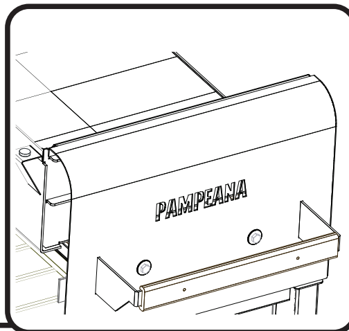
Fig 4 : insertar los tornillos dentro de la cavidad y dejar reposar el lateral haciendo coincidir frente y base de la ménsula con el filo de chapa. No lleva tuerca en esta sujeción.
